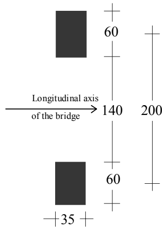
Fig. 16. Load model n. 2 (single axle)
