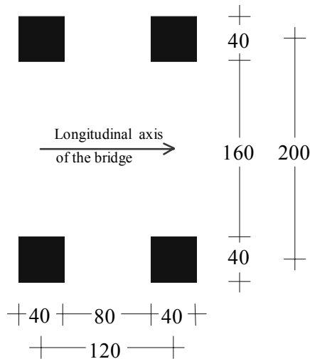
Fig. 14. Tandem system
