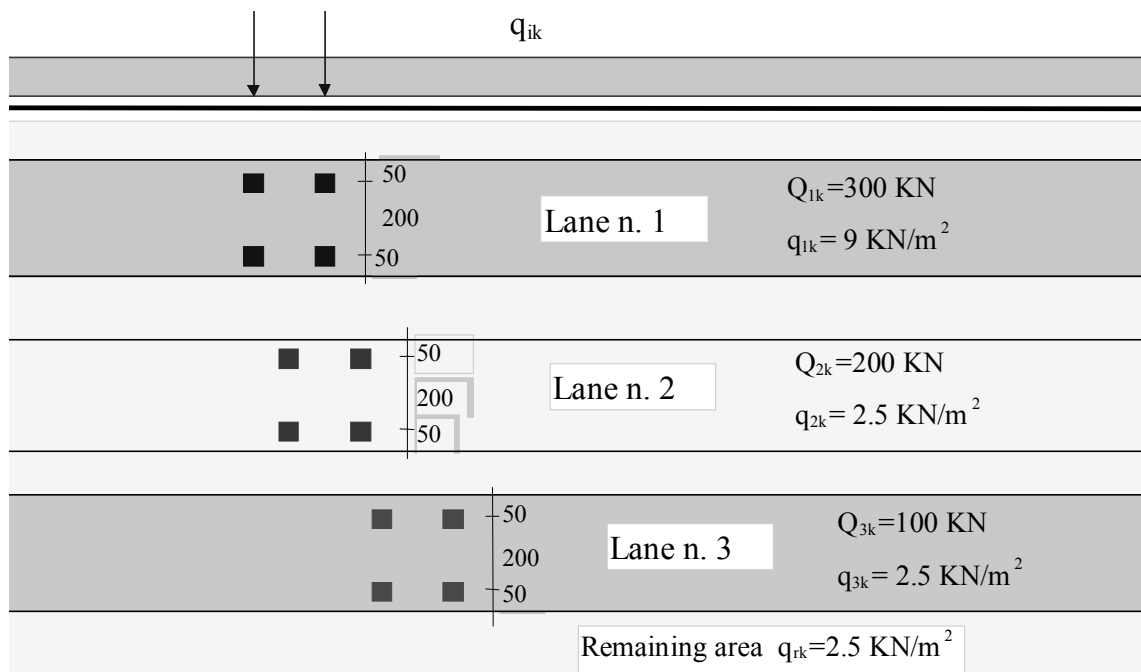
Fig. 15. Example of application of the load model n.1
